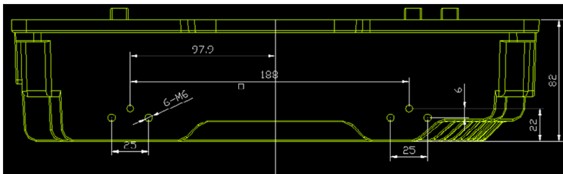
图 5 室外固定台安装孔位图
