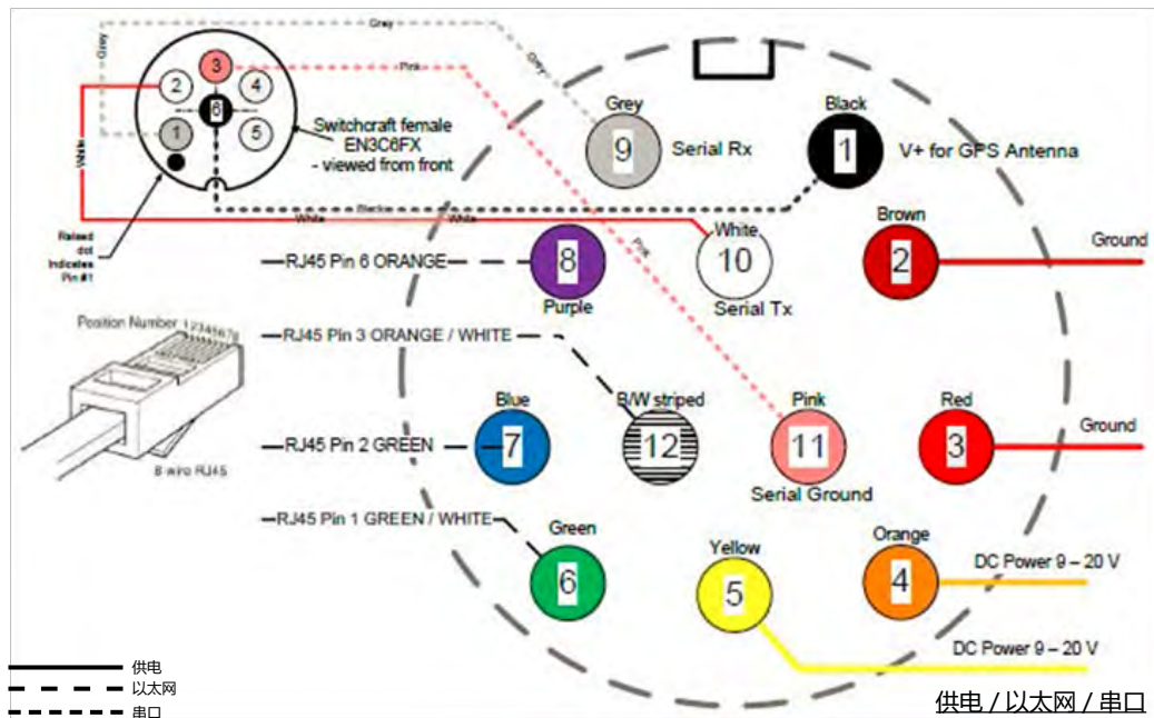
图 1 供电（可选）/ 串口 / 以太网引脚说明图（接线端）
