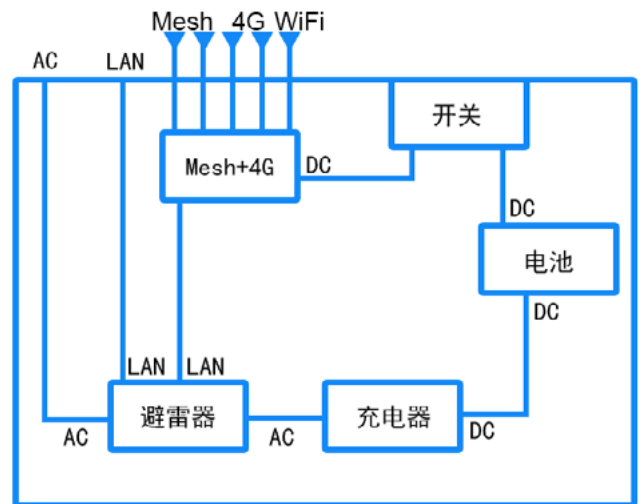
内部连接示意图
