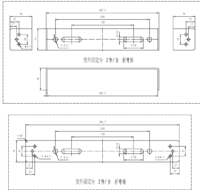
图 4 室外固定台内部孔位图
