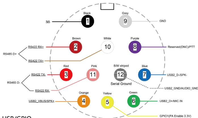
图 2 AUX 引脚说明图 (接线端)
