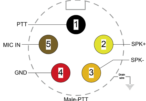
图 3 PTT 引脚说明图 (接线端)
