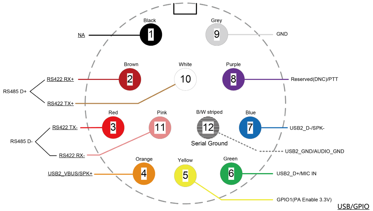
图 2 USB/GPIO 引脚说明图（接线端）
